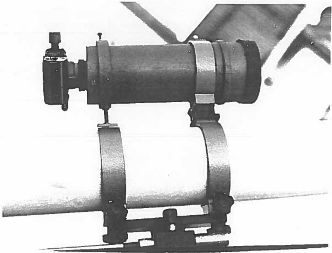
Detalle del acople para la astrocámara de 80mm F/3 . La caja portapelícula es de una legendaria Werlisa Color, de la cual solo queda el nombre. La versión definitiva permitirá utilizar una cámara reflex normal.
